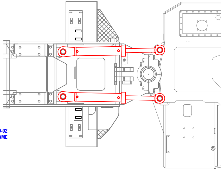
M350-201-02 REAR FRAME
